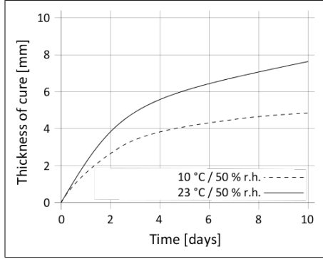
Діаграма 1: Швидкість полімеризації Sikaflex®-529 Evolution
